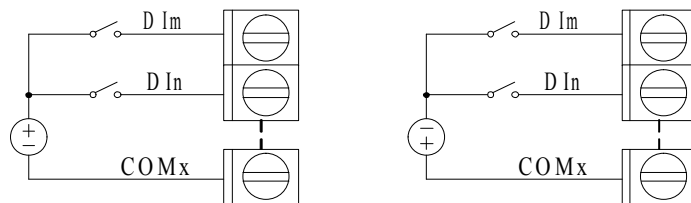
图 3.5 开关信号输入
