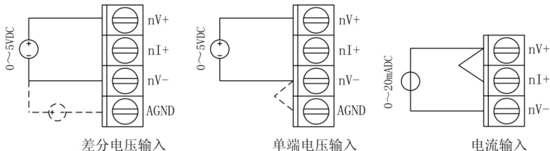
图 3.4 模拟信号输入
