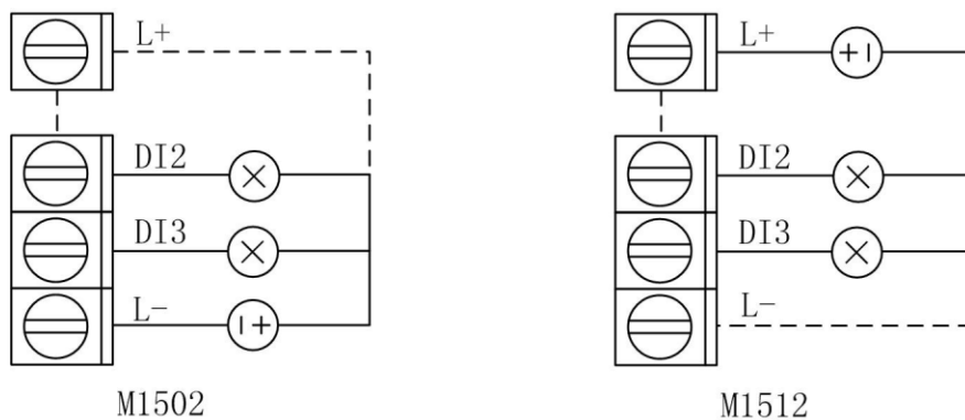
图 3.6 开关信号输出
