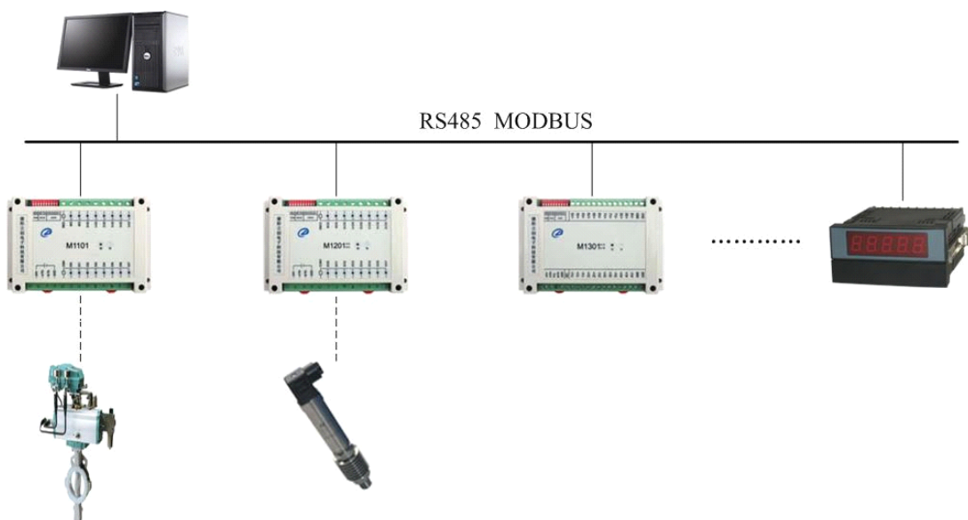
图 6.1 M1502 应用示例
