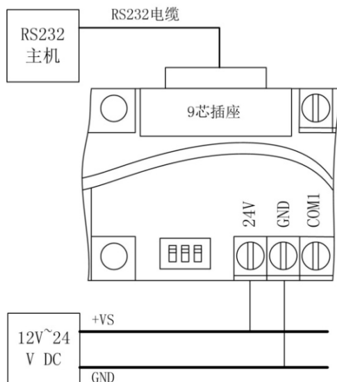
图 3.3 RS232 总线模块电源和通讯线连接
