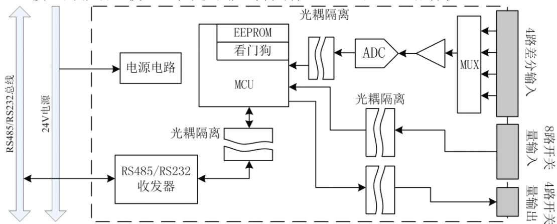
图 1.1 M1502/12 原理框图
