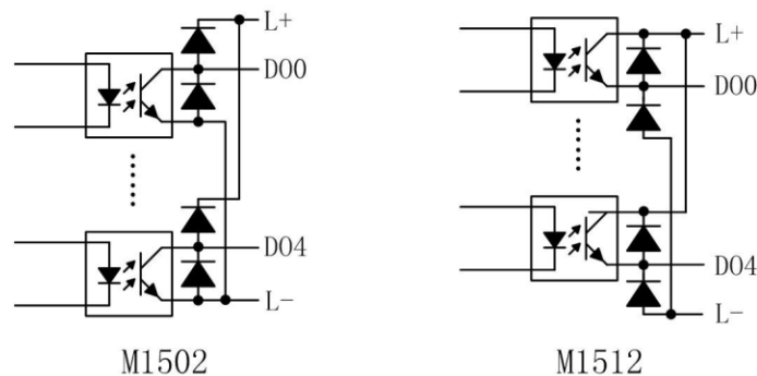
图 2.3 开关量输出电路
