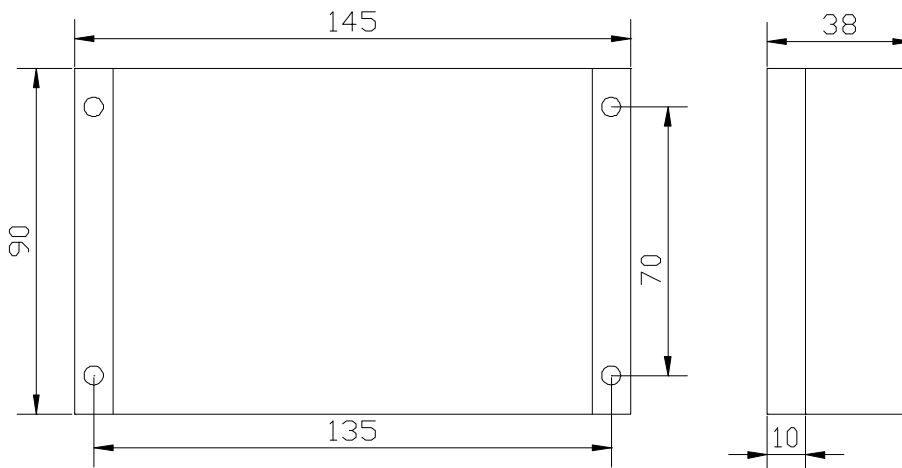
图 1.3 模块尺寸
