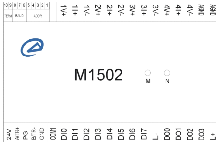
图 3.6 M1502/12 端子与拨码开关排列
