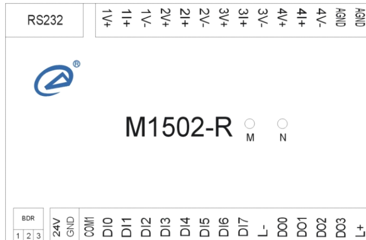
图 3.7 M1502/12-R 端子与拨码开关排列
